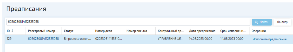
Рис. 4 Строка поиска
